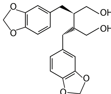
Dihidrocubebina
