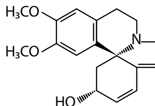
Eritravina
